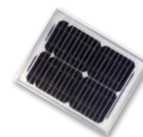
Solarmodule voor Novomatic 423 Accu uitvoering Vermogen Pmax: 10Wp Nominale spanning: 21.5V Stroom bij Pmax:a 0,5A Afmetingen: 370 x 310 mm 4,1 kg
